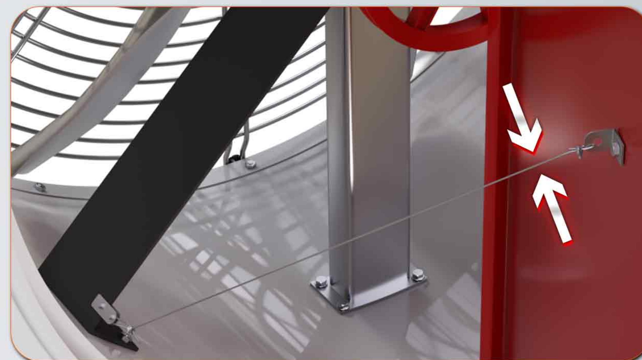
مکانیزم محدود کننده دمپر
